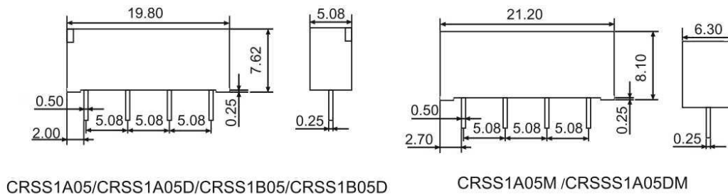
外形尺寸图 Dimensions
